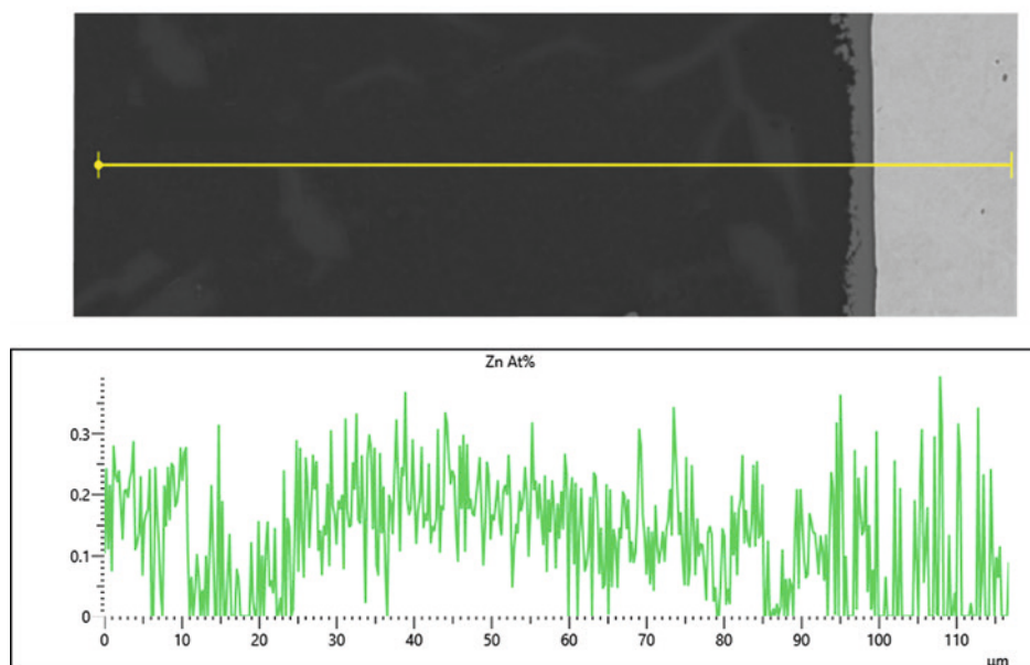
Bild 4: Querschliff durch die Interdiffusionszone eines ursprünglich mit 100 µm feuerverzinkten Inserts aus Stahl 1.4571 mit Aluminiumlegierung AlSi9Mg nach Sandguss bei 780°C. REM-Bild (oben) sowie der zugehörige EDX-Linescan mit der Elementinformation für Zink (unten).
