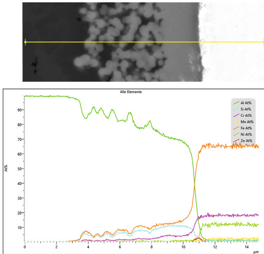
Bild 3: Querschliff durch die Interdiffusionszone eines ursprünglich mit 100 µm Schichtdicke feuerverzinkten Inserts aus Stahl 1.4571 mit der Aluminiumlegierung AlSi9Mg nach Sandguss bei 740°C. REM-Bild (oben) in hoher Vergrößerung und Darstellung der Elementinformation mittels EDX-Linescan für alle Elemente (unten). Zink ist nur in geringer Konzentration und in einem sehr engen Schichtdickenbereich zwischen 10,6 und 11,4 µm detektierbar.
