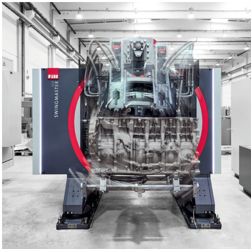
Abb.1: Entkernmaschine SWINGMASTER 500
