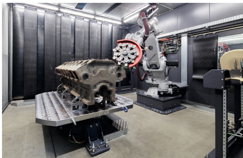
Abb.3: Roboter Schleifmaschine GRIND PERFORMER im Fill Testcenter
